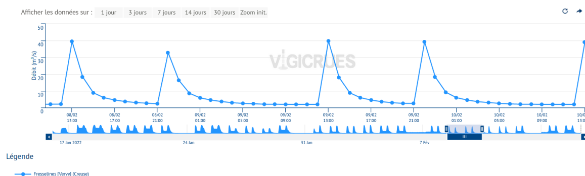
Figure 22: Hydrogrammes à Aubusson et Fresselines montrant les variations de débits générées par les barrages hydroélectriques de l'axe Creuse (source : vigiecrue)
