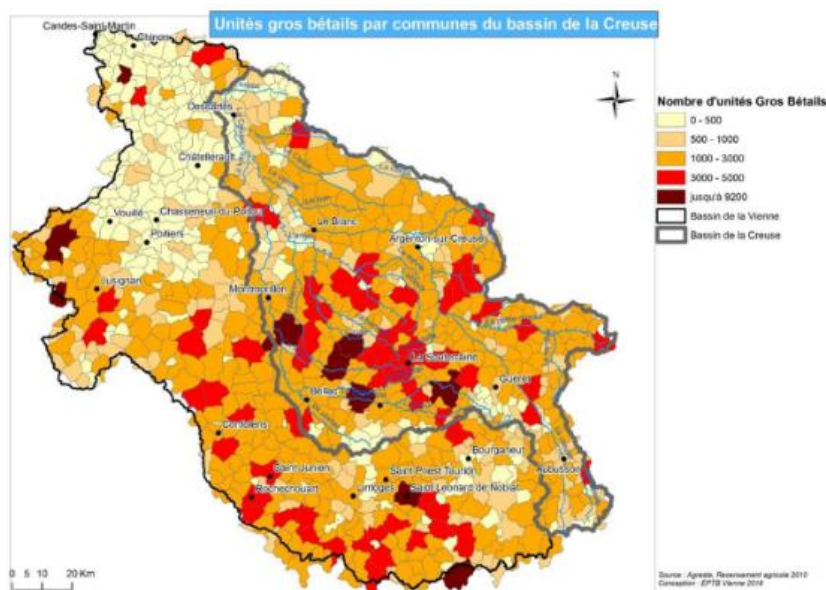
Figure 17: Unités gros bétails (UGB) par commune sur le bassin de la Creuse (1 UGB correspond à une vache adulte)
