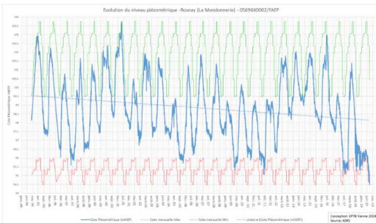
Figure 18: Evolution du niveau piézométrique à Rosnay
