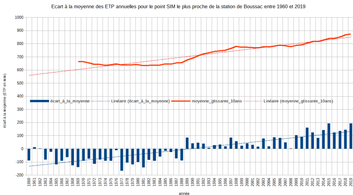
Figure 15: Ecart à la moyenne des évapotranspirations annuelles pour la station de Boussac entre 1960 et 2019
