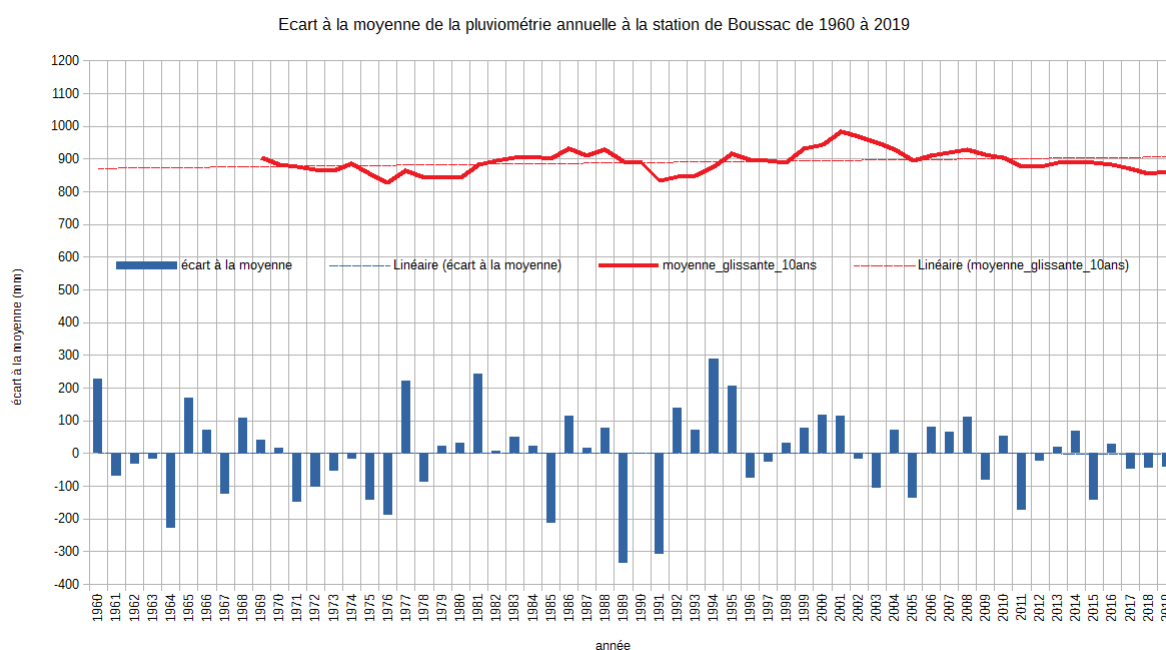
Figure 14: Ecart à la moyenne de la pluviométrie annuelle à la station de Boussac de 1960 à 2019
