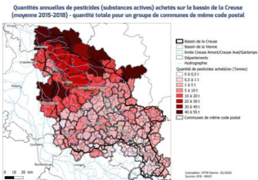
Figure 23: quantités annuelles de pesticides achetées sur le bassin de la Creuse par groupe de communes
